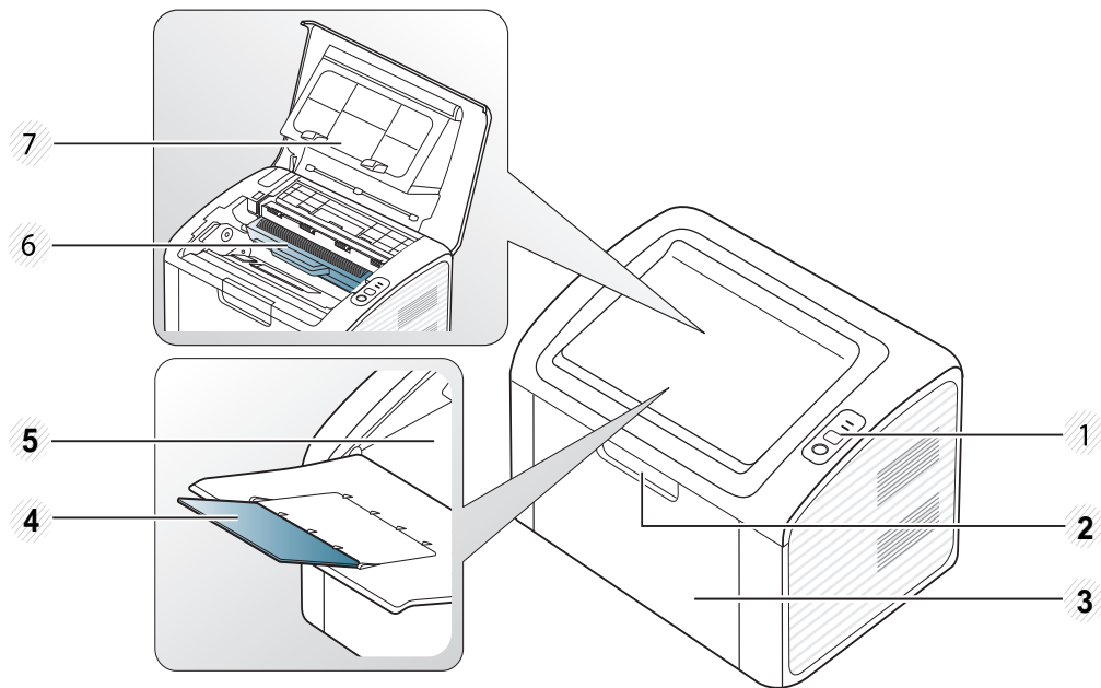
正视图
